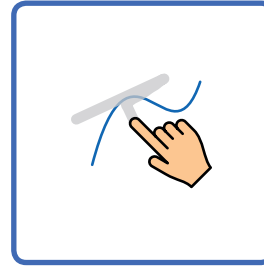
Styczna do wykresu
