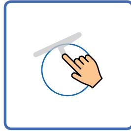
Styczna do okręgu
